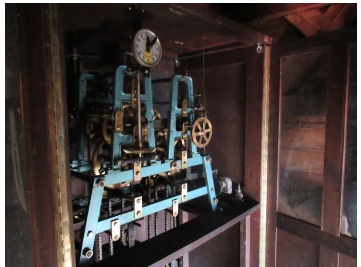
Věžní hodiny
