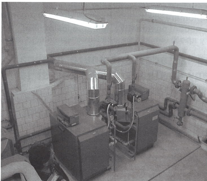
KOTELNA
